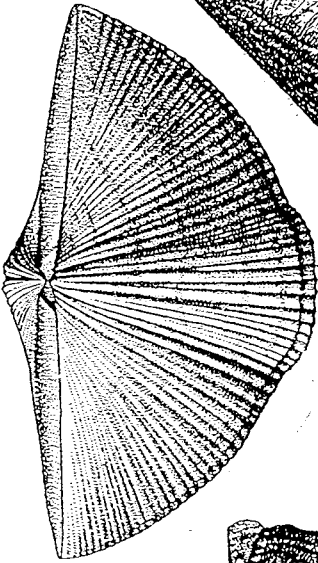
brachiopoden
