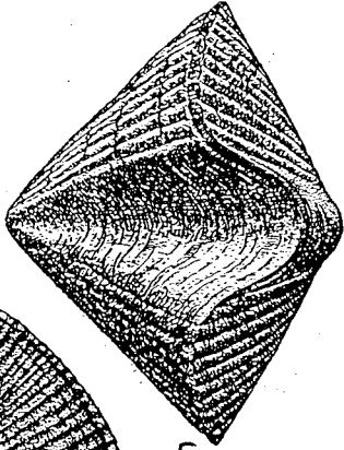
brachiopoden
