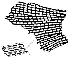
mosdiertjes
