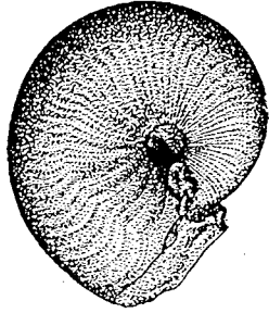
ammoniet
