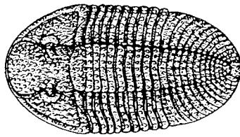
trilobiet
