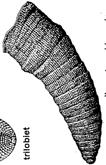
alleenstaand koraal
