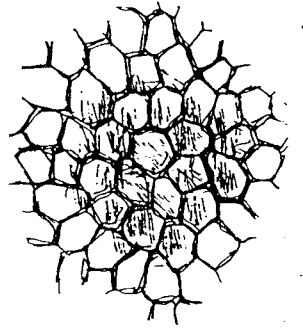
honingraatkoraal
